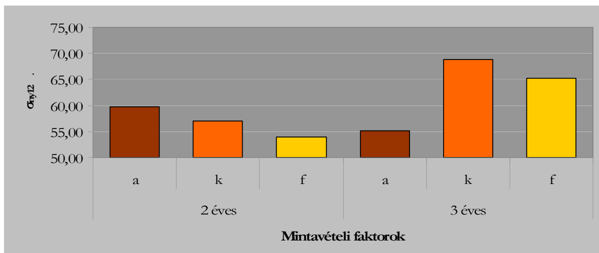
69. ábra – A próbatestek faktorok szerinti nyomószilárdsága (Amerika 10) [MPa]
