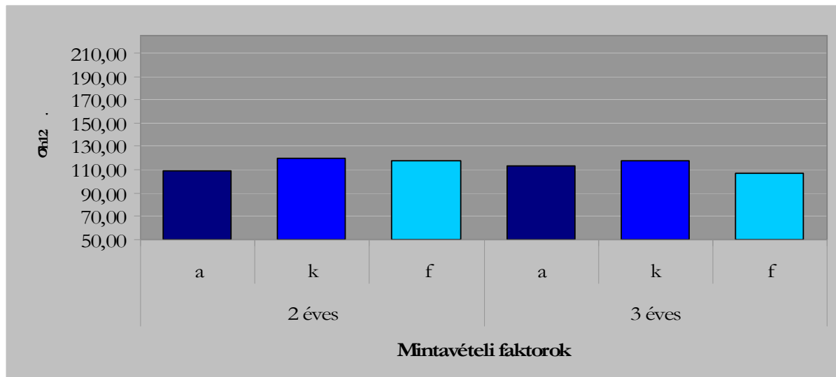
75. ábra – Zempléni minták faktorok szerinti hajlítószilárdsága [MPa]
