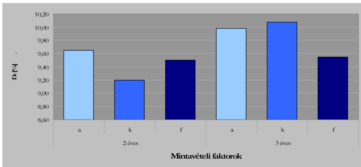
39. ábra – A zalai származású minták húrirányú dagadása [%] az érlelési idő és rakatszint függvényében
