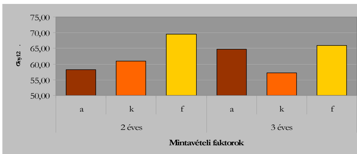
66. ábra – A próbatetek faktorok szerinti nyomószilárdsága (somogy) [MPa]
