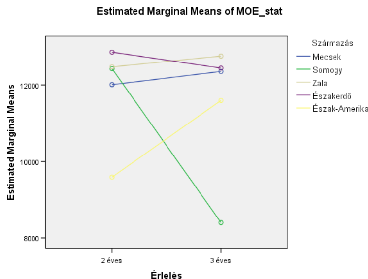
85. ábra – Az érlelési idő és a hajlítószilárdság kapcsolata
