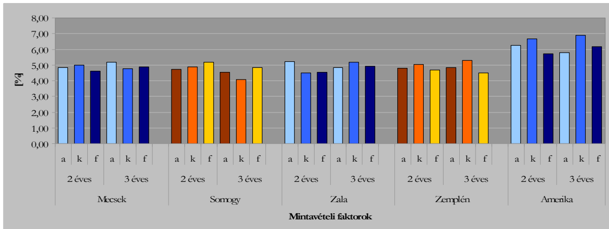
58. ábra – Származási hely, érlelési idő és a rakatban elfoglalt szint szerinti sugár irányú dagadás [%]
