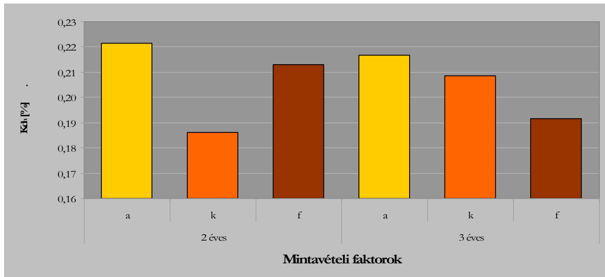
42. ábra - A zempléni származású minták dagadási együtthatója az érlelési idő és rakatszint függvényében
