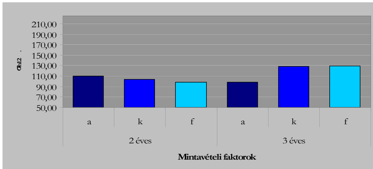
76. ábra – Amerikai minták faktorok szerinti hajlítószilárdsága [MPa]
