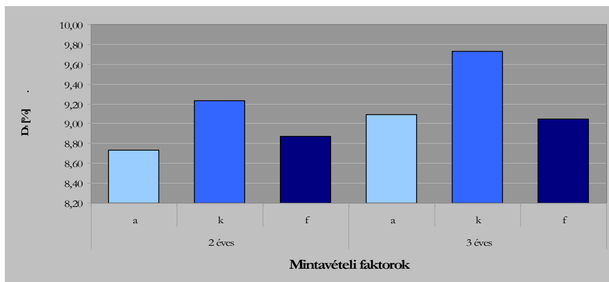
43. ábra – Az amerikai származású minták húrirányú dagadása [%] az érlelési idő és rakatszint függvényében
