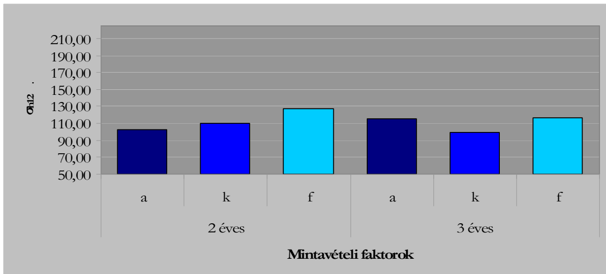
73. ábra – Somogyi minták faktorok szerinti hajlítószilárdsága [MPa]
