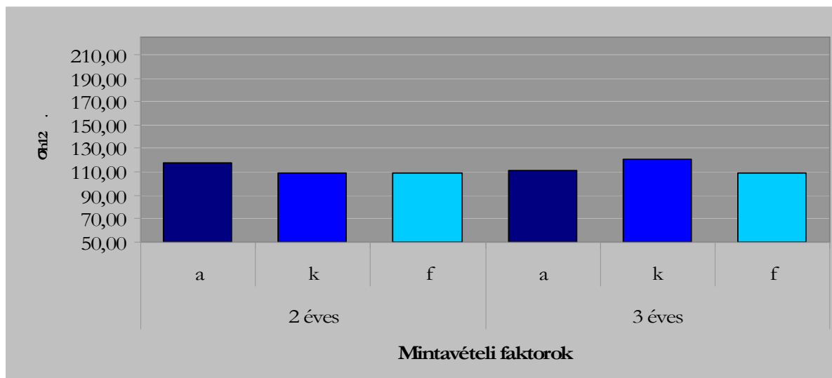
74. ábra – Zalai minták faktorok szerinti hajlítószilárdsága [MPa]
