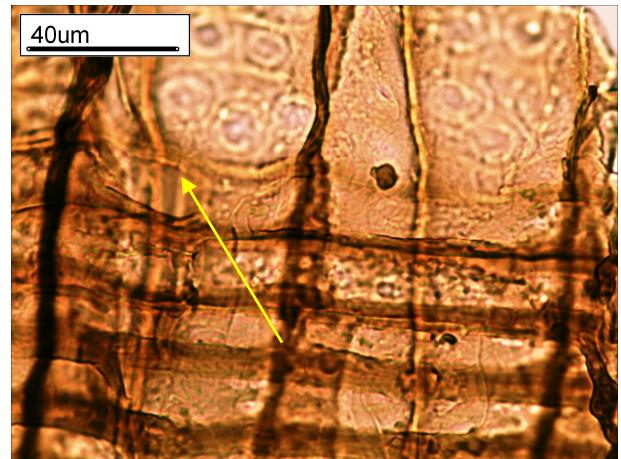
46. ábra A bélsugar heterogén felépítésű (6-os minta)
