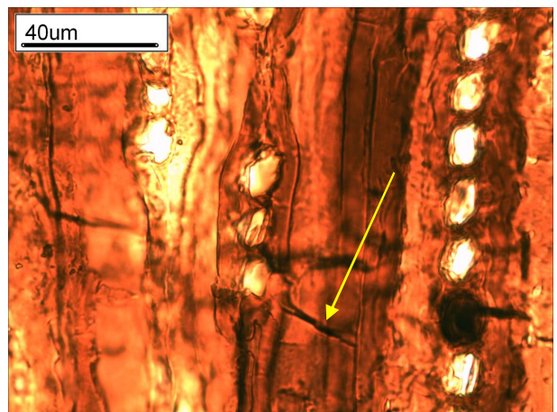
82. ábra A hosszparenchima harántfala sima (13-as minta)
