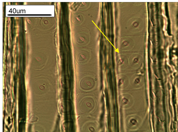
88. ábra Az udvarosgödörkék 1-2 sorban láthatóak ( Taxodium distichum )
