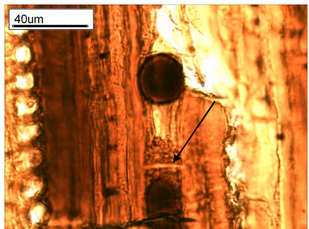
55. ábra A hosszparenchima harántfala sima (7-es minta)
