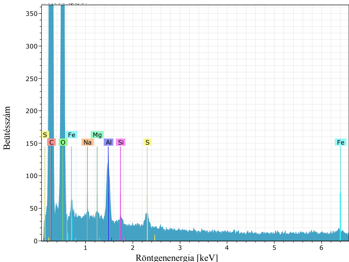
21. ábra Az 5-ös törzs, ősi Taxodioxylon germanicum röntgenspektruma
