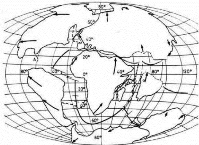
111. ábra A földrészek helyzete a kréta korban
