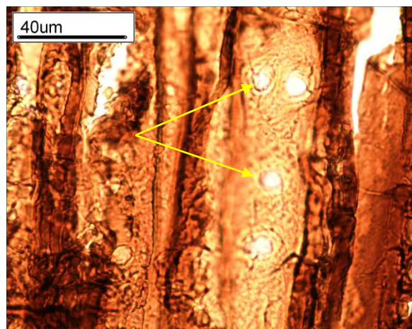
79. ábra Udvaros gödörkék 1-2 sorban (13-as minta)
