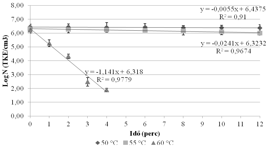
11. ábra: A Zygosaccharomyces bailii NCAIM Y.00954 T túlélő sejtjeinek száma modell közegben hőkezelve
