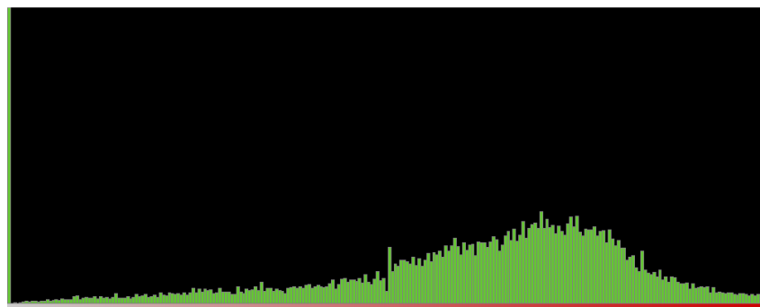
22. ábra A tesztkép S értékeinek eloszlása
